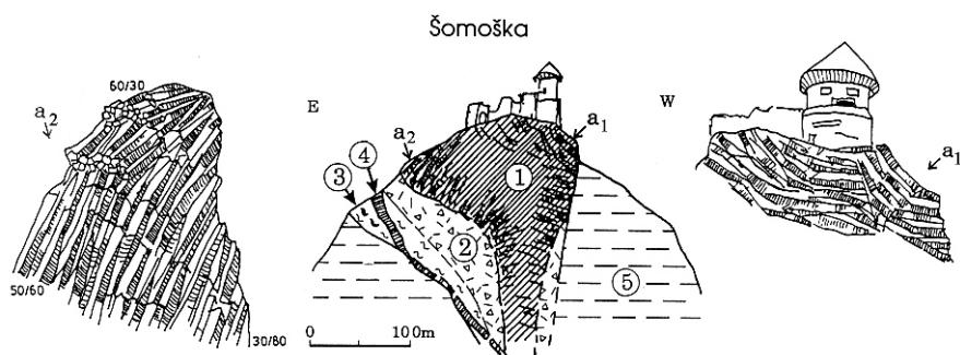
Lokalita č. 41 Šomoška (E 4). Schéma stavby bazaltového neku a diatrémy: 1 - bazaltový nek, a1 - stĺpcová odlučnosť pri západnom okraji neku, a2 - stĺpcová odlučnosť pri východnom okraji neku; 2 - tufy a brekcie vo výplni diatrémy; 3 - bazaltové trosky pri okraji diatrémy; 4 - bazaltová dajka; 5 - spodnomiocénne sedimenty.
